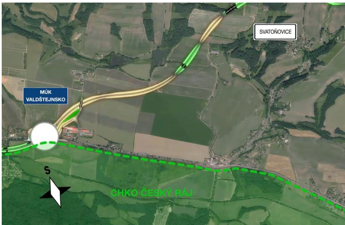
Obr. 44: Výřez z vizualizace Valbek pro ŘSD se zákresem CHKO Český ráj a plánované přeložky silnice I. třídy I/35.
